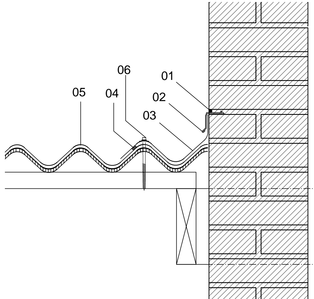
Lodret snit - Tilslutning skorsten
