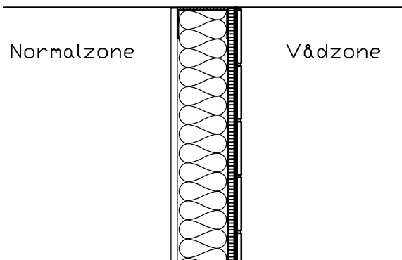
Lodret snit - Tilslutning til loft 1:10
